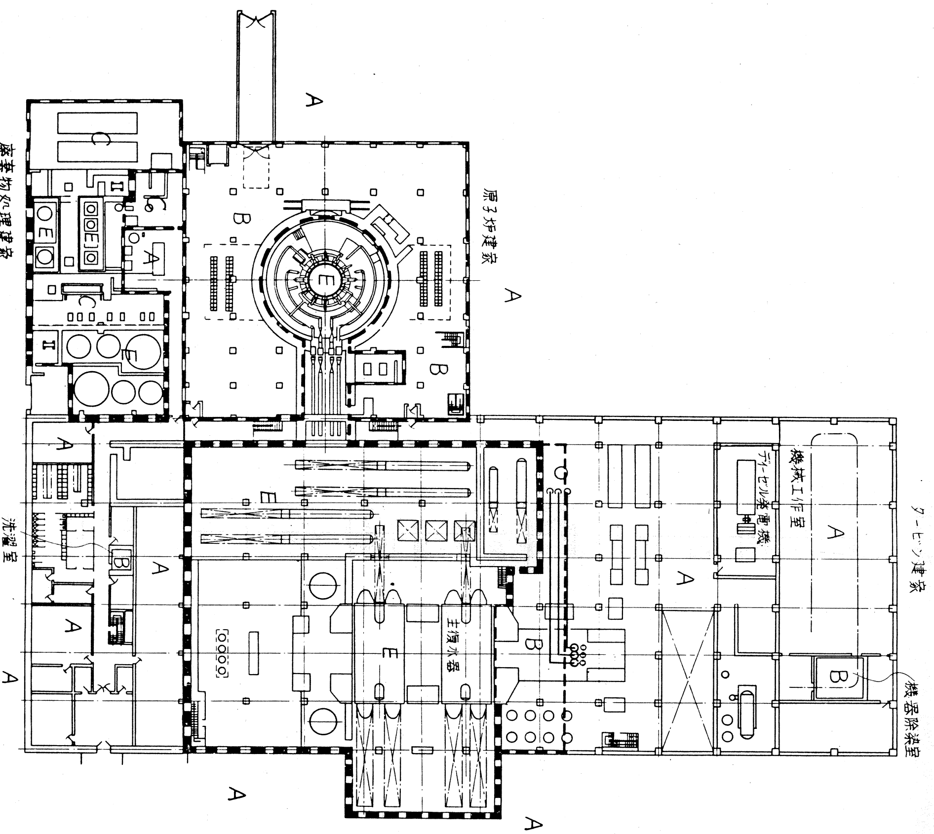
第92-2図 1)の設計上の区域区分(1階平面)
