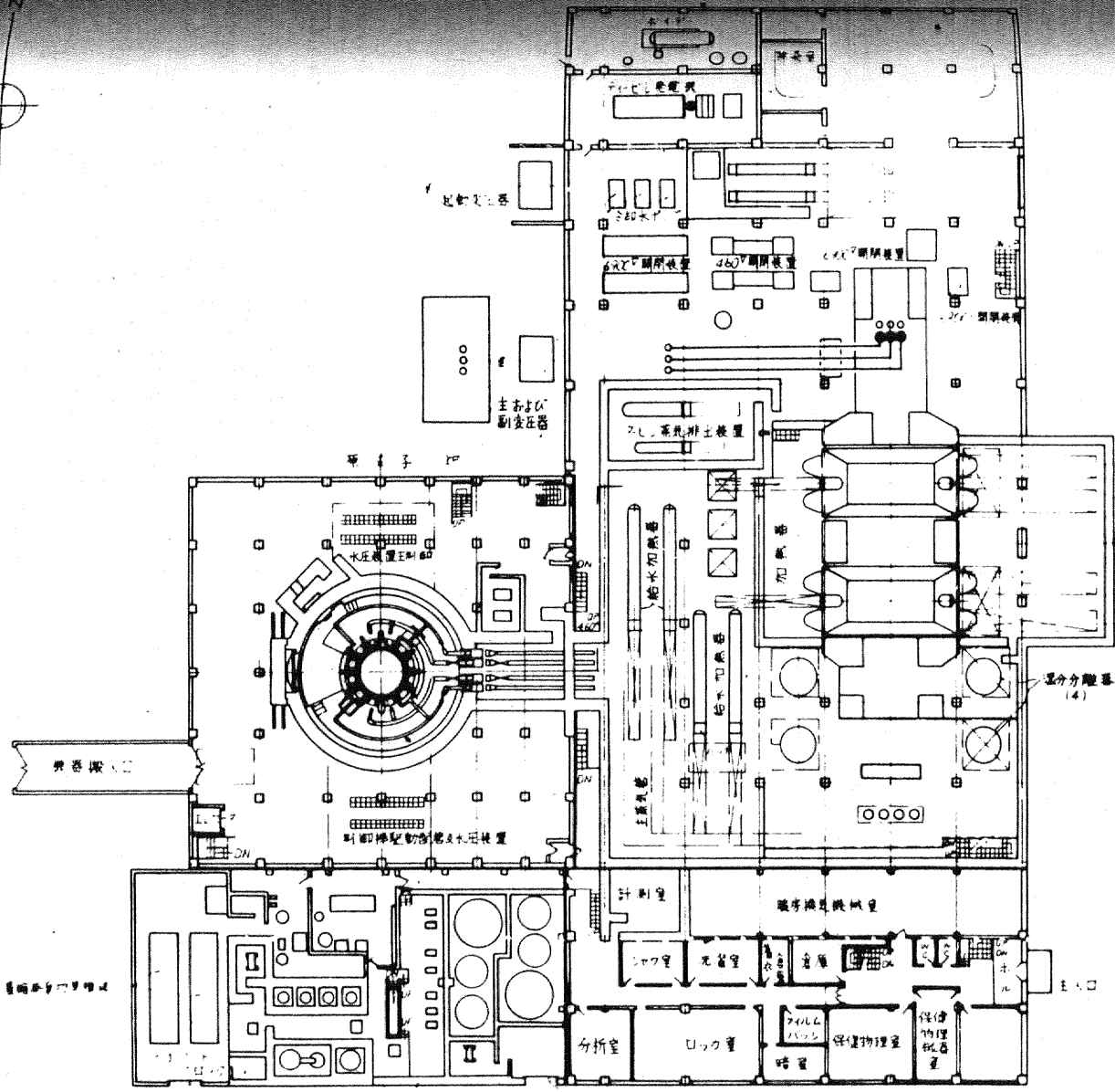
第2.1-2図 一階平面図
